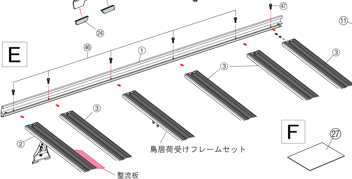
構成部品
