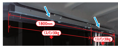
▲装着例：RW-16N / NV350キャラバン・バン/標準ルーフ・ロングボディ
