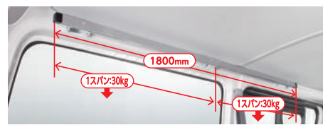
▲装着例：RW-16 / 200V系ハイエース・バン/標準ルーフ・標準ボディ
