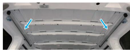
▲装着例：RW-16V / NV200バネット・バン
