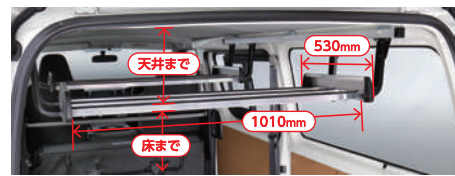
▲装着例：RW-10 / 200V系ハイエース・バン (2台装着時 / 3台同時装着可能)
